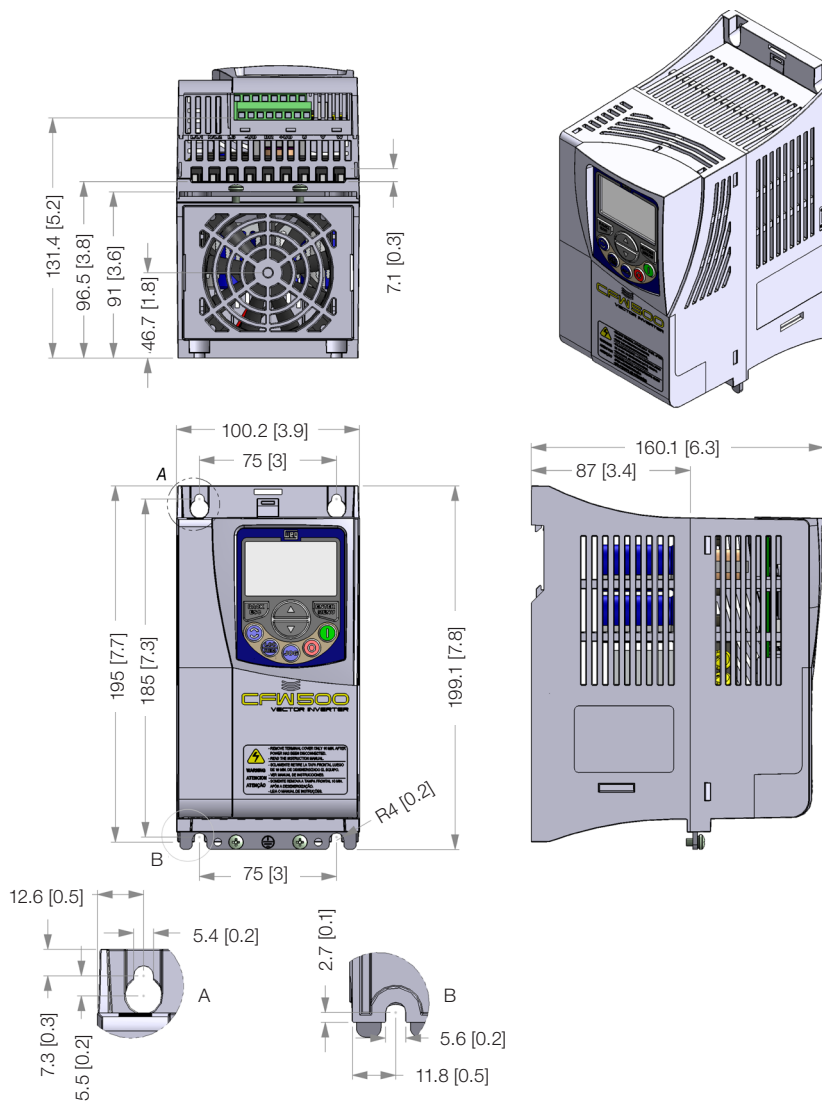
Figure B.5: Inverter di mensions in mm [in] – frame B Figura B.5: Dimensiones del convertidor de frecuencia en mm [in] – mecánica B Figura B.5: Dimensões do inversor em mm [in] – mecânica B
