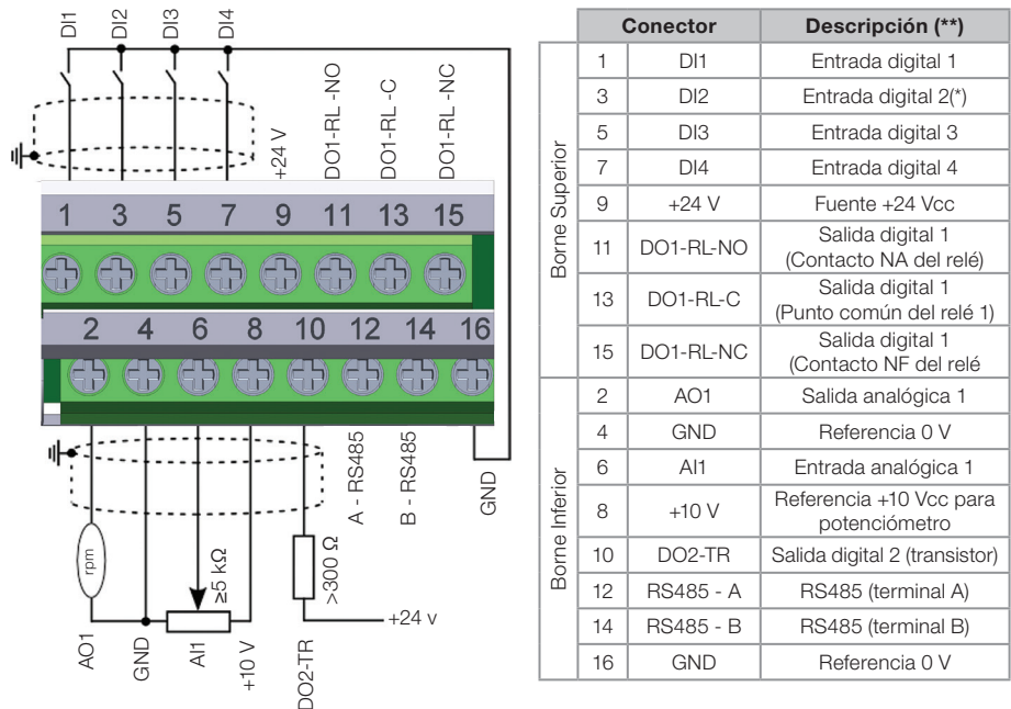
Figura 3.4: Señales del conector del módulo plug-in CFW500-IOS
