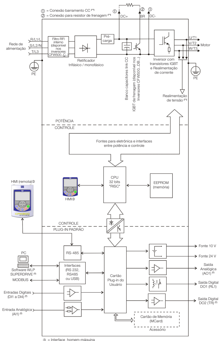
Figura 2.1: Blocodiagrama do CFW500
