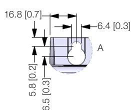
Figure B.6: Inverter dimensions in mm [in] – frame C Figura B.6: Dimensiones del convertidor de frecuencia en mm [in] – mecánica C Figura B.6: Dimensões do inversor em mm [in] – mecânica C
