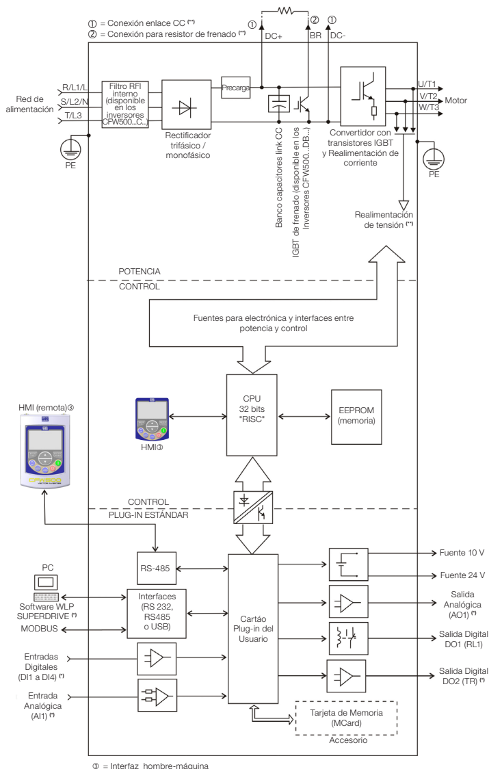
Figura 2.1: Diagrama de bloques del CFW500
