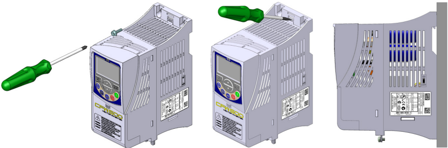
(a) Surface mounting (a) Montaje en superficie (a) Montagem em superfície (b) DIN Rail Mounting (b) Montaje en riel DIN (b) Montagem em trilho DIN
