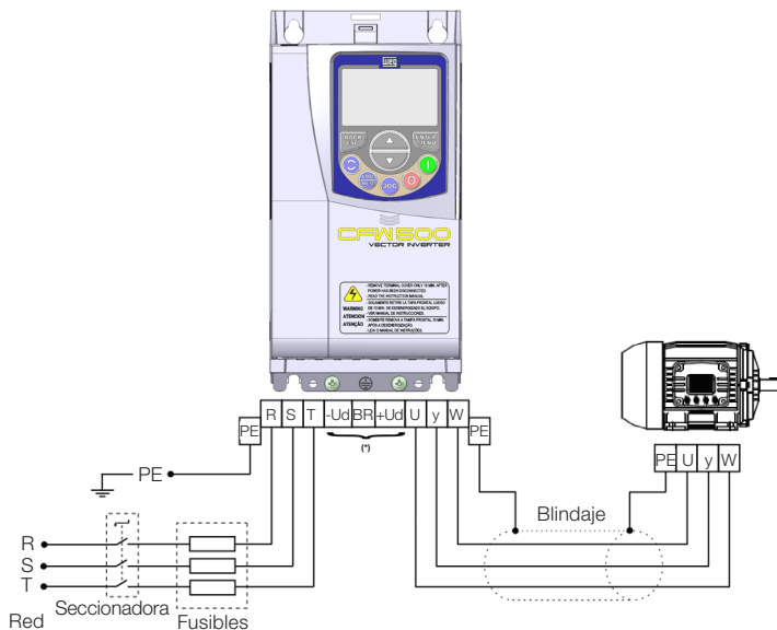
Figura 3.1: Conexiones de potencia y aterramiento
