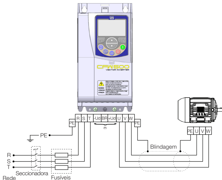
Figura 3.1: Conexões de potência e aterramento
