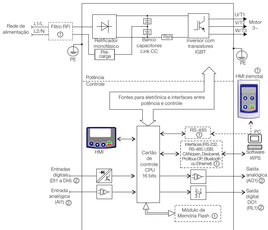
Figura 2.2: Blocodograma do CFW300 para mecânica A 110 V
