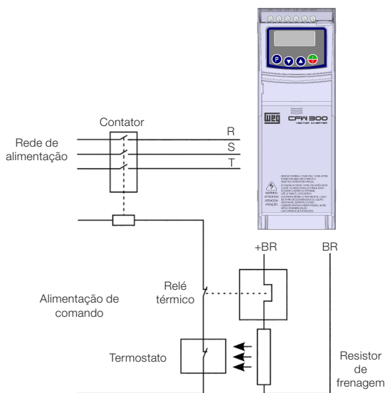
Figura 3.2: Conexão do resistor de frenagem
