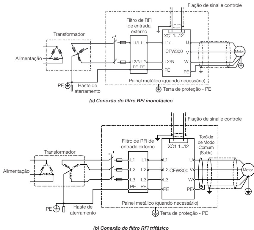
Figura 3.5: (a) e (b) Conexão do filtro supressor de RFI - condição geral
