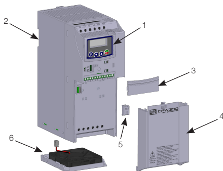
Frame size C / Tamanho C / Mecânica C
