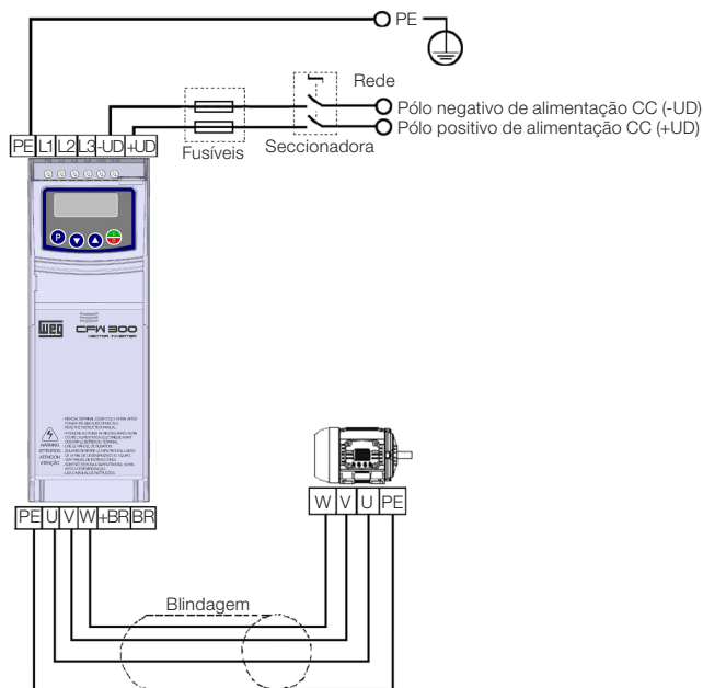
(c) Mecânicas B e C alimentação CC
