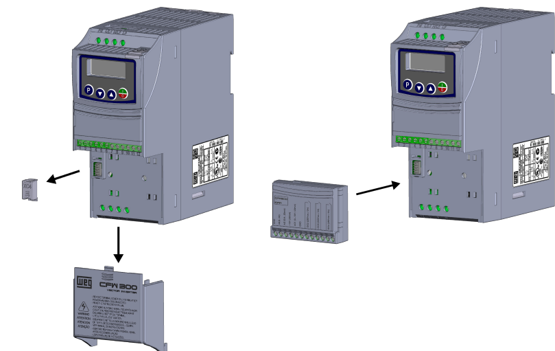
(a) Removal of the protection cover of the connection of the IO expansion accessory (a) Remoción de la tapa de protección de la conexión de los accesorios de expansión de IOs (a) Remoção da tampa de proteção da conexão dos acessórios de expansão de IO's
