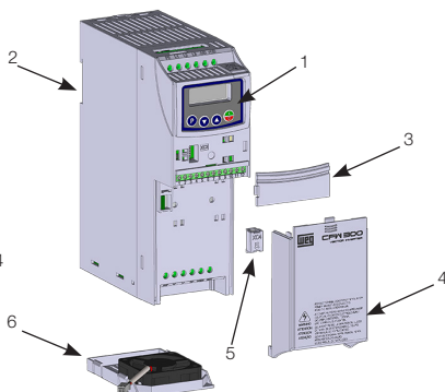
Frame size C / Tamanho C / Mecânica C
