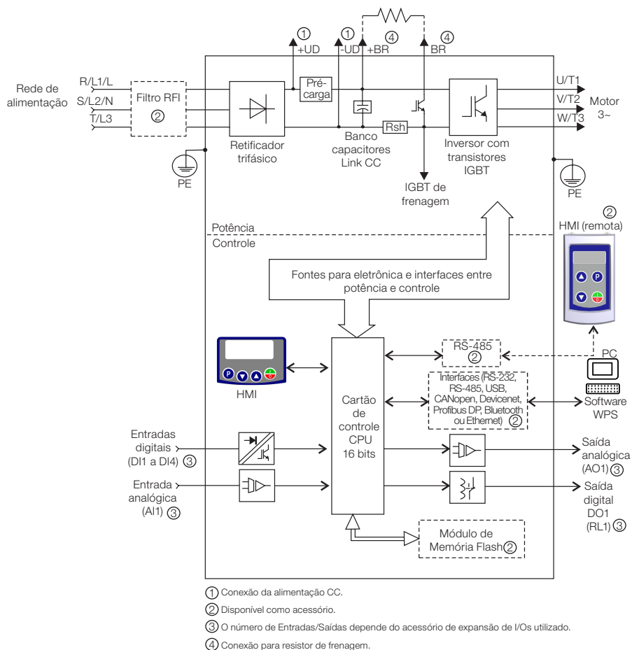
Figura 2.3: Blocodograma do CFW300 para mecânica B 220 V
